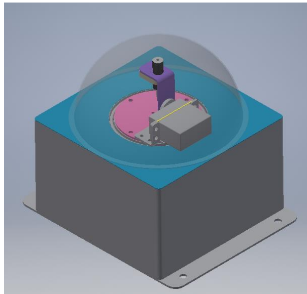
两轴激光指示云台
